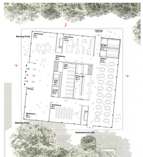
Grundriss
